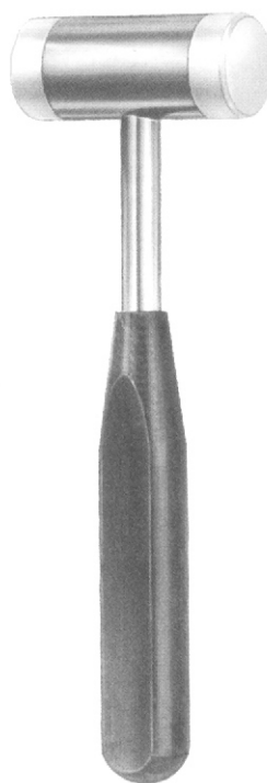
VF-77-3970 19 cm/7 1/2" Ø 25 mm 300 g
